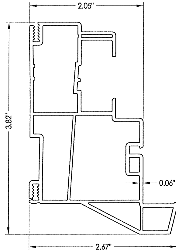
3 JAMB
