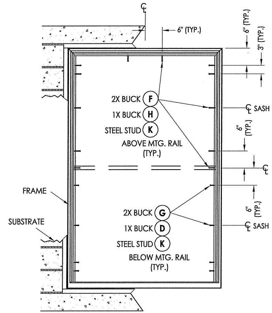
FRAME ANCHORING 1X/2X/STEEL STUD
